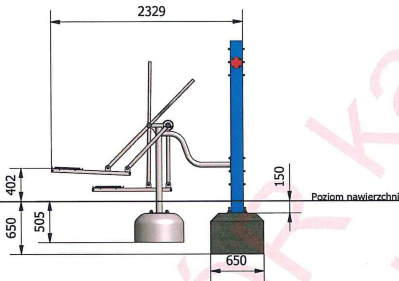
WIDOK 1
