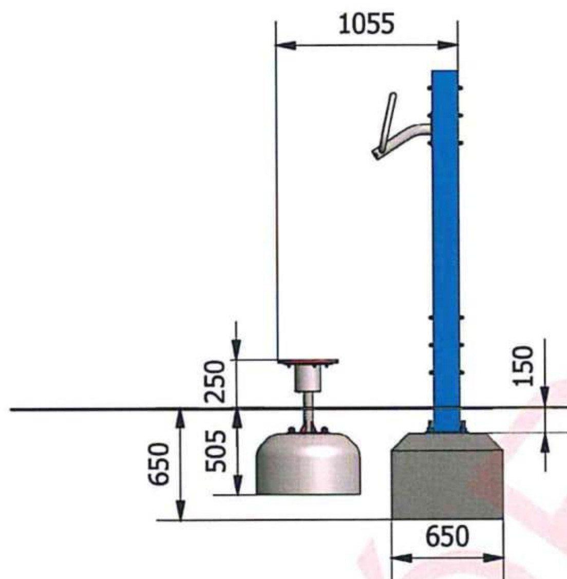
WIDOK 1
