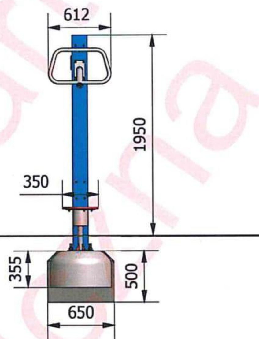
WIDOK 2
